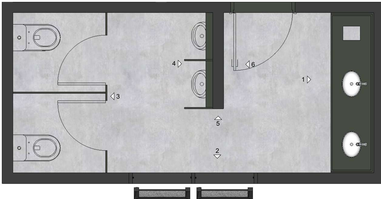
WC MASCULINO PLANTA BAIXA ESC: 1/25
