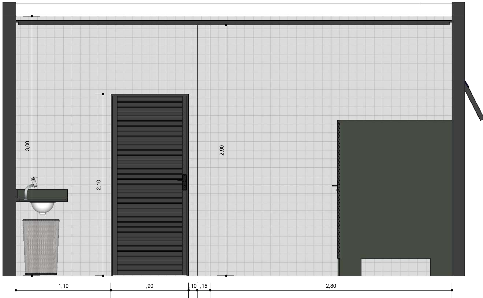
WC FEMININO VISTA 3 ESC: 1/25
