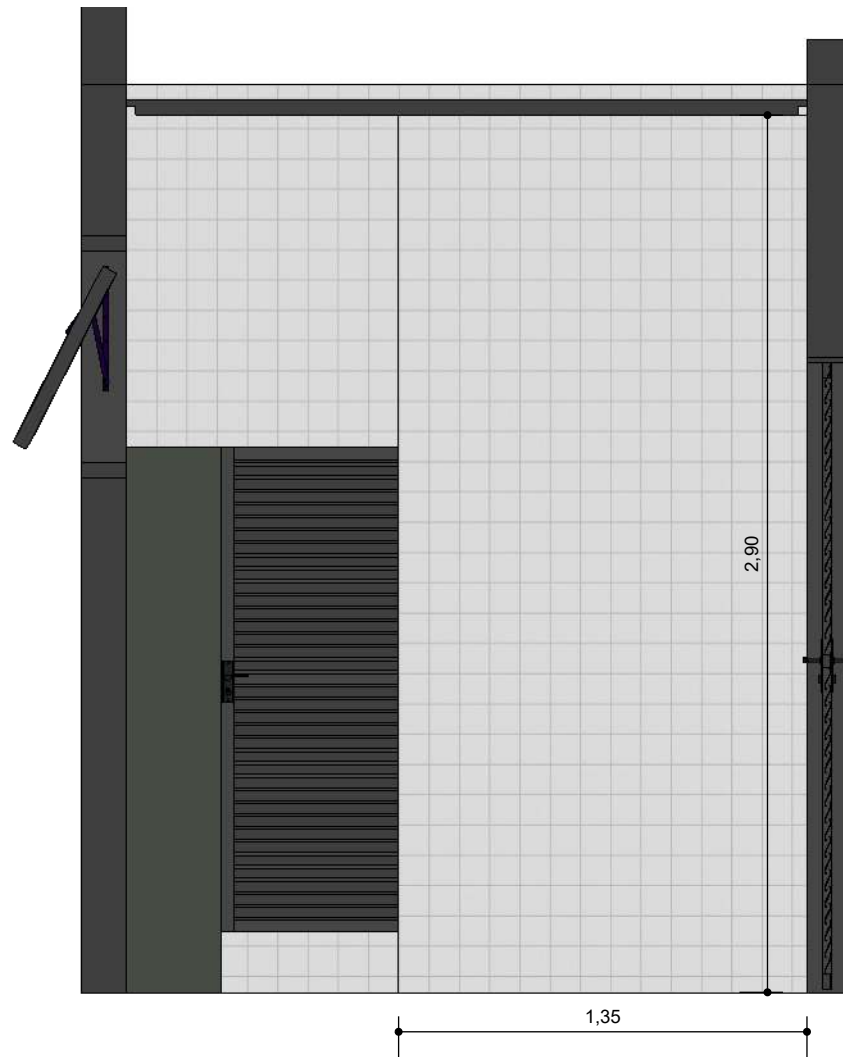
WC MASCULINO VISTA 6 ESC: 1/25
