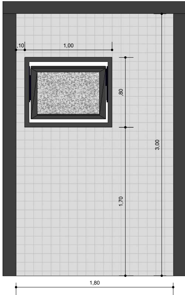
WC PNE VISTA 3 ESC: 1/25
