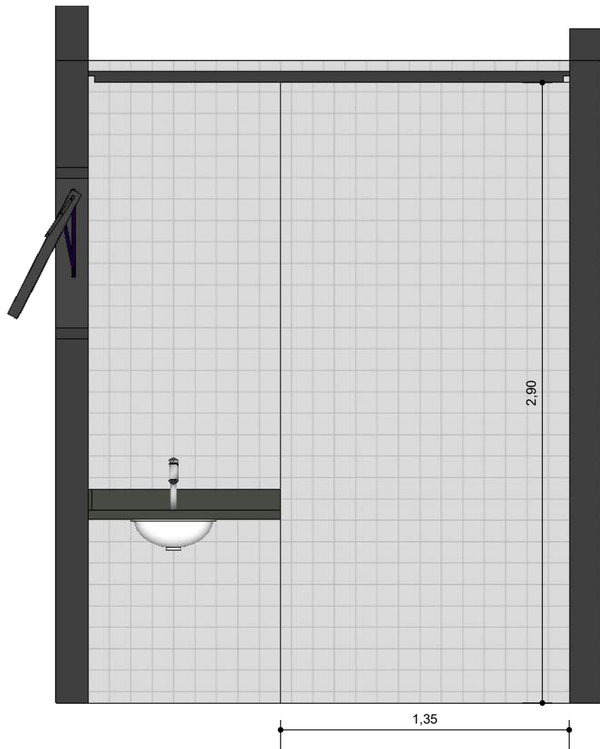
WC FEMMININO VISTA 4 ESC: 1/25
