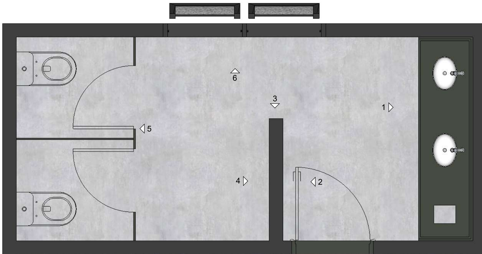
WC FEMININO PLANTA BAIXA ESC: 1/25
