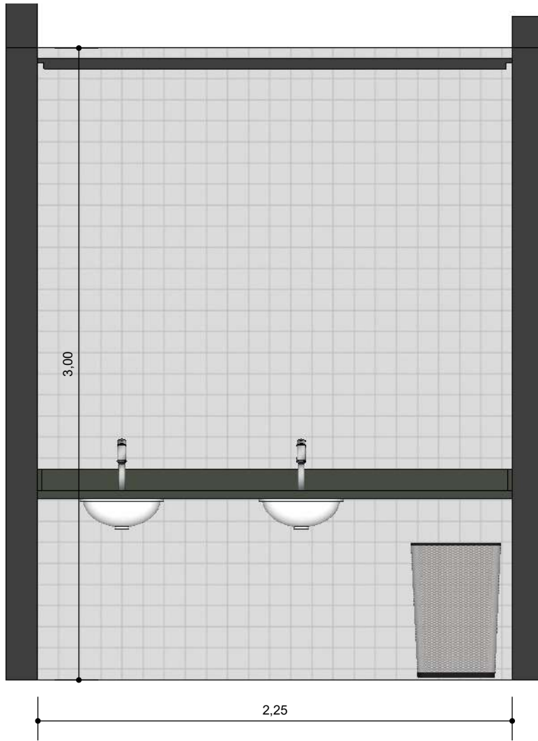
WC FEMININO VISTA 1 ESC: 1/25
