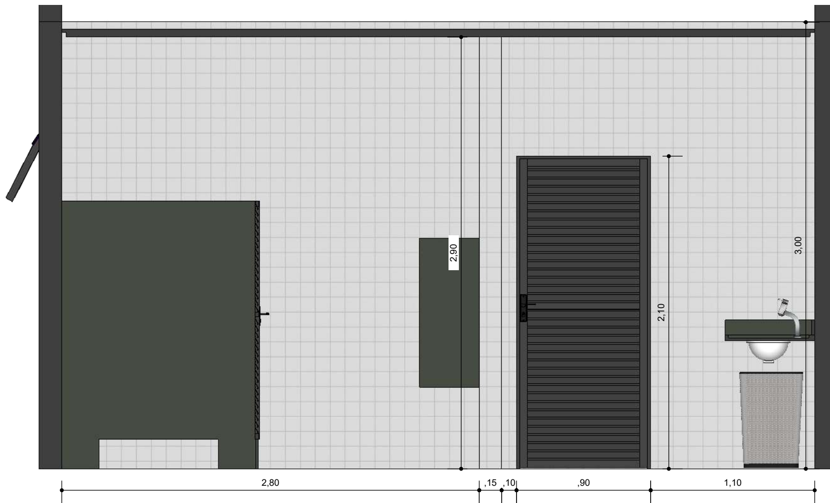
WC MASculINO VISTA 5 ESC: 1/25
