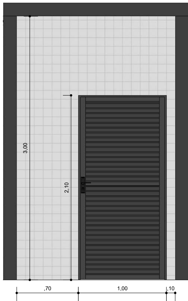
WC PNE VISTA 1 ESC: 1/25
