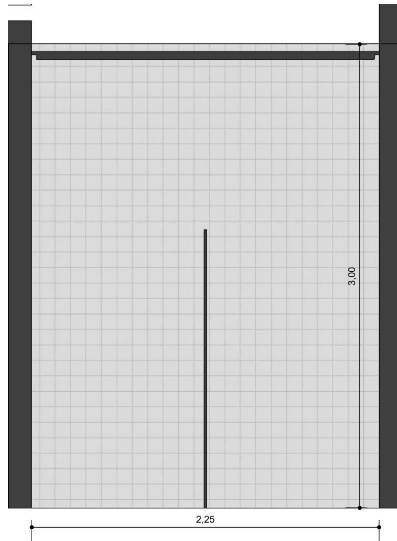
WC FEMMININO VISTA 5 ESC: 1/25
