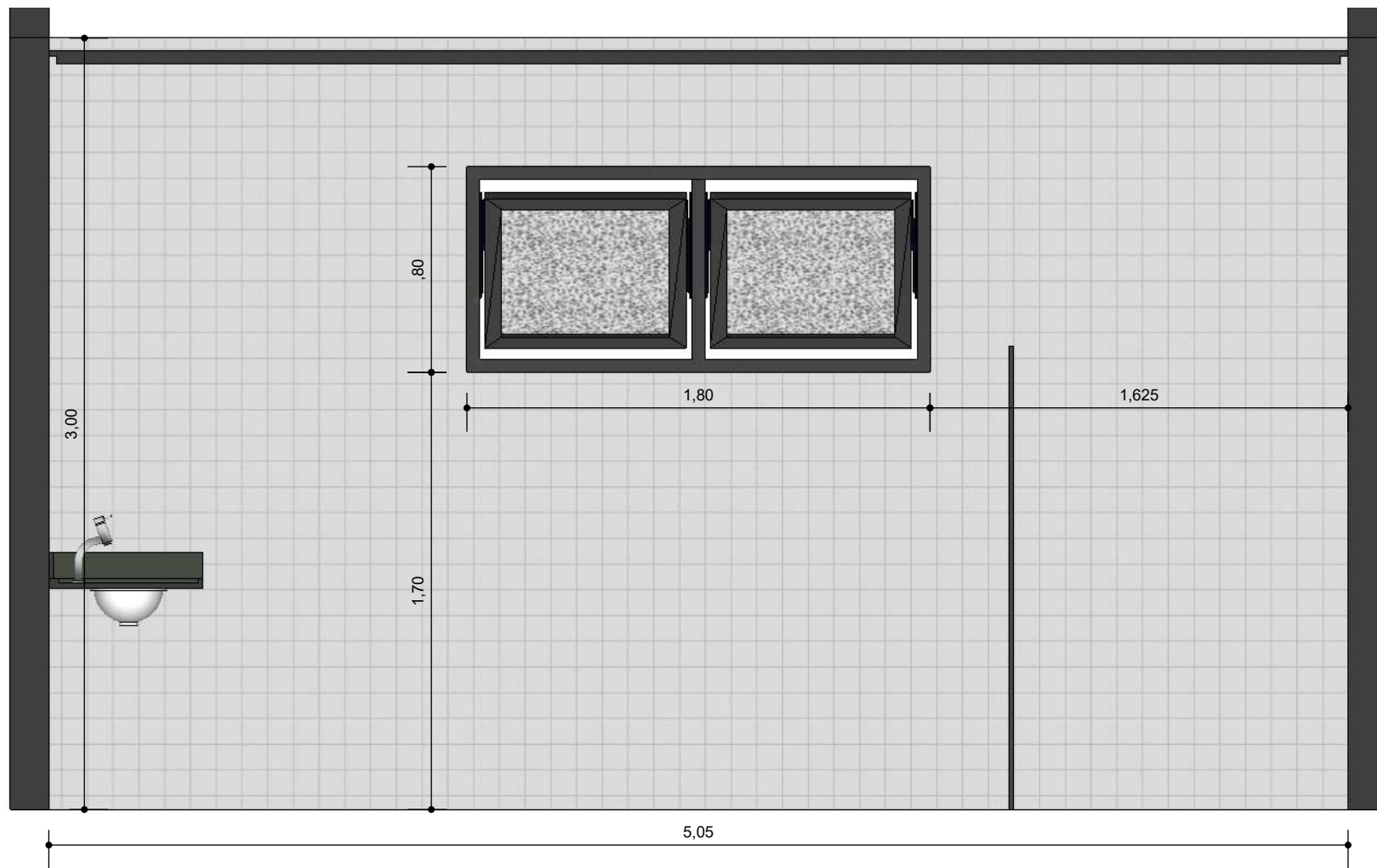
WC MASCULINO VISTA 2 ESC: 1/25
