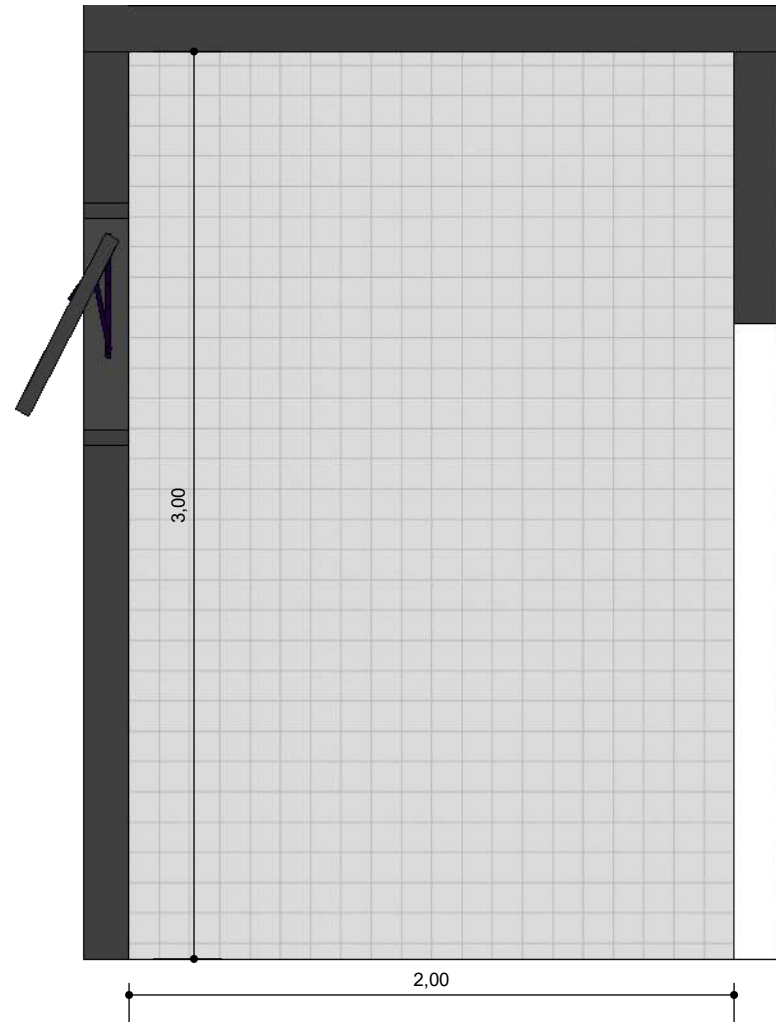
WC PNE VISTA 4 ESC: 1/25
