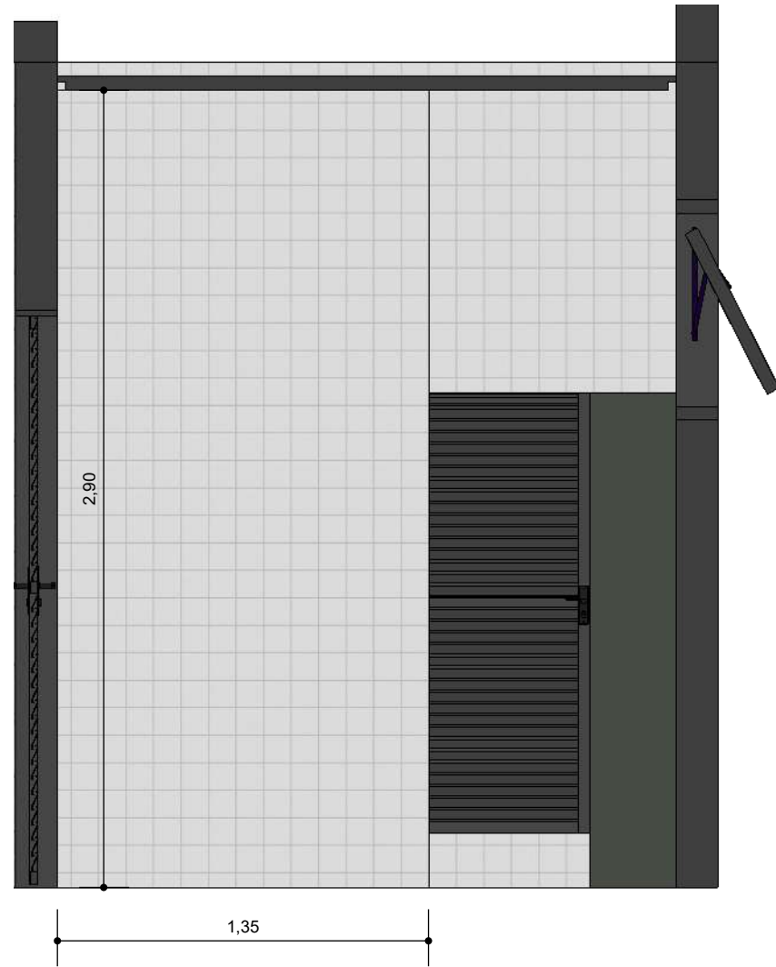
WC FEMININO VISTA 2 ESC: 1/25
