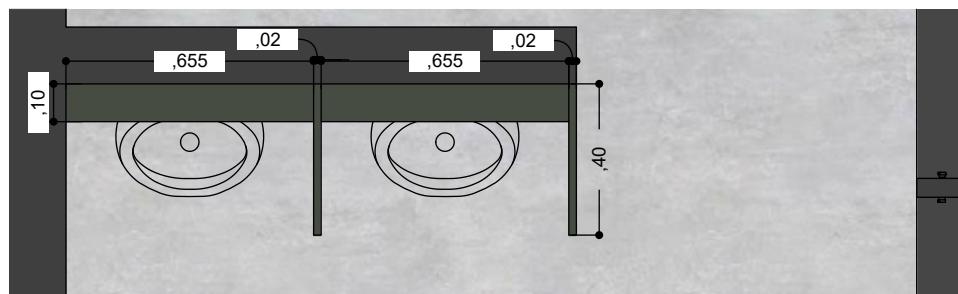
WC MASCULINO - DIVISÓRIAS MICTÓRIO PLANTA BAIXA / ESC: 1/20
