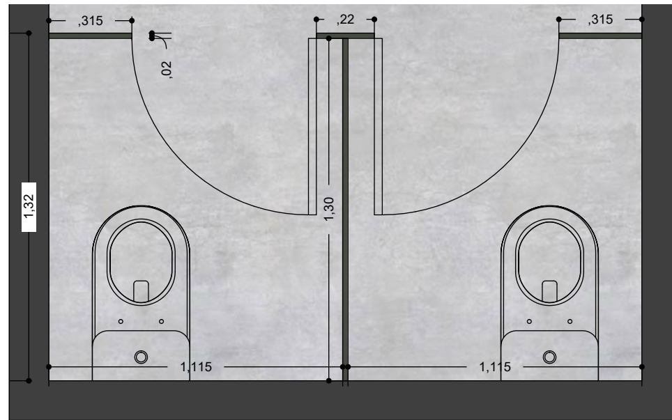
WC FEM. E MAS. - DIVISÓRIAS PLANTA BAIXA / ESC: 1/20
