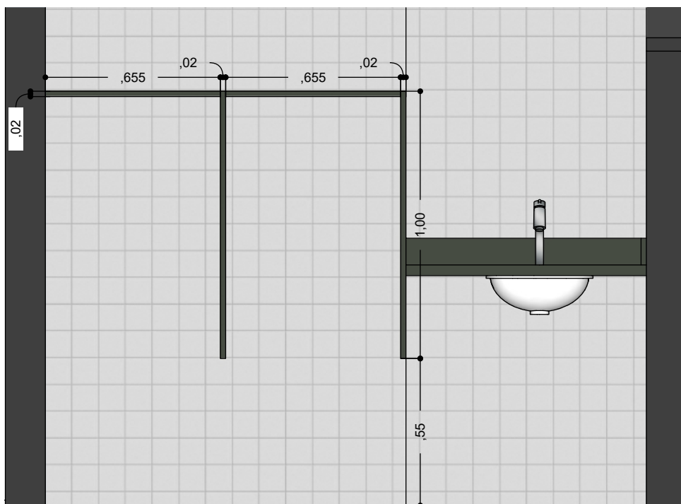
WC MASCULINO - DIVISÓRIAS MICTÓRIO VISTA FRONTAL / ESC: 1/20
