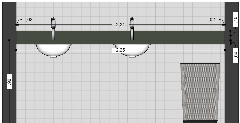
WC FEMININO VISTA FRONTAL ESC: 1/20
