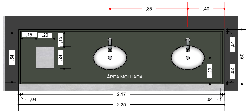
WC MASCULINO - BANCADA PLANTA BAIXA ESC: 1/20
