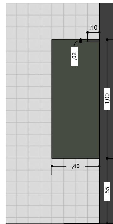
WC MASCULINO - DIVISÓRIAS MICTÓRIO VISTA LATERAL / ESC: 1/20
