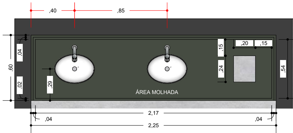
WC FEMININO - BANCADA PLANTA BAIXA ESC: 1/20
