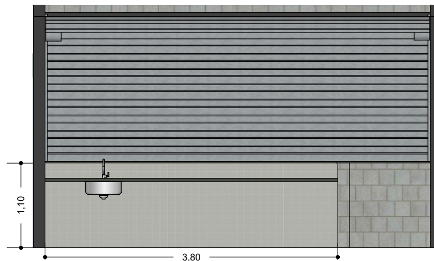
VISTA 3 ESC: 1/50
