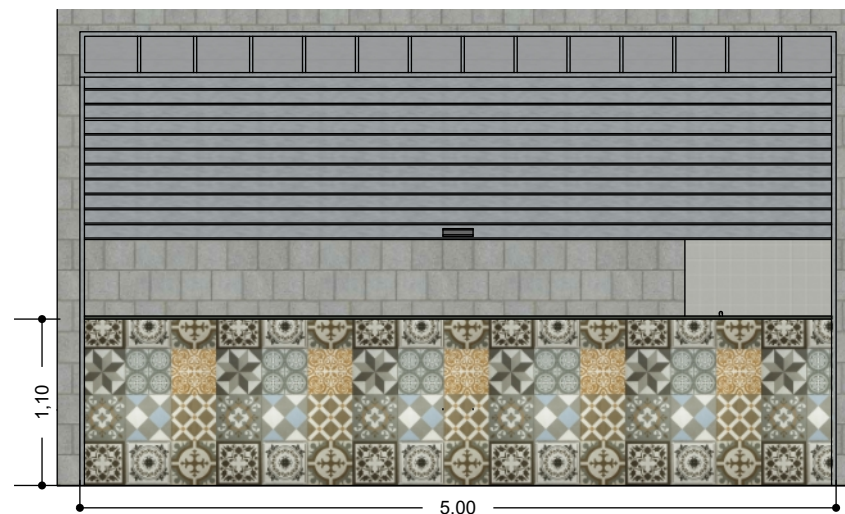
VISTA 1 ESC: 1/50
