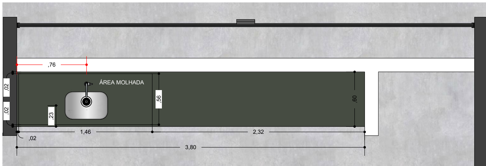
BAR - BALCÃO INFERIOR PLANTA BAIXA ESC: 1/25
