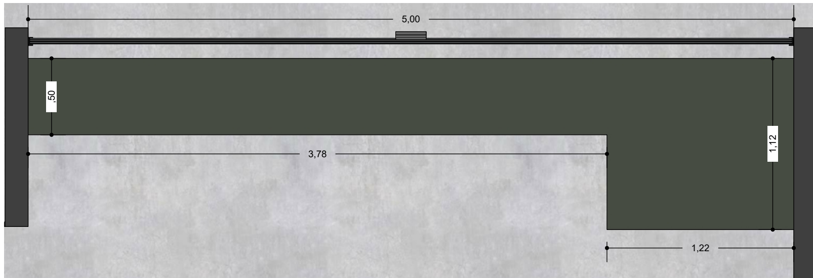
BAR - BALCÃO SUPERIOR PLANTA BAIXA ESC: 1/25
