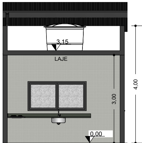
CORTE A-A ESC: 1/75
