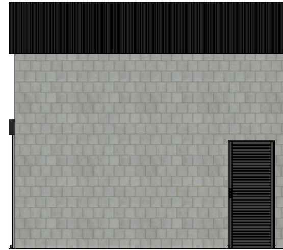
ELEVAÇÃO 01 ESC: 1/100
