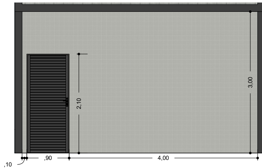
VISTA 1 ESC: 1/50
