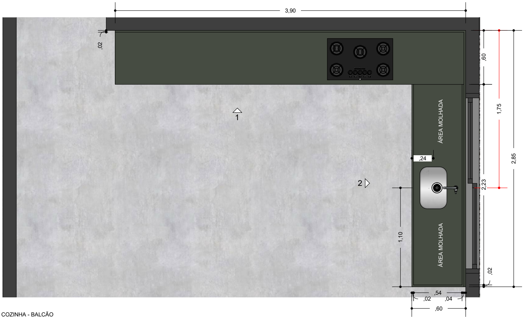
COZINHA - BALCÃO PLANTA BAIXA ESC: 1/25
